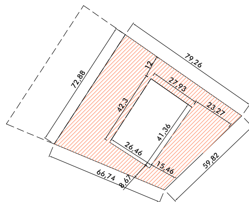
AREA DE MOVIMIENTO PLANTA SOTANO Y SEMISOTANO
