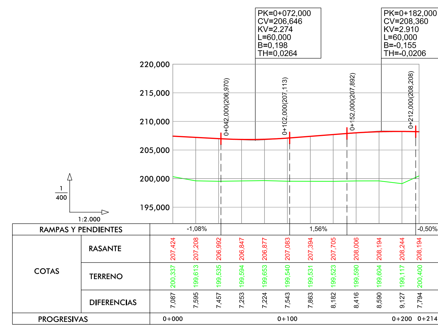
PERFIL LONGITUDINAL EJE 4b
