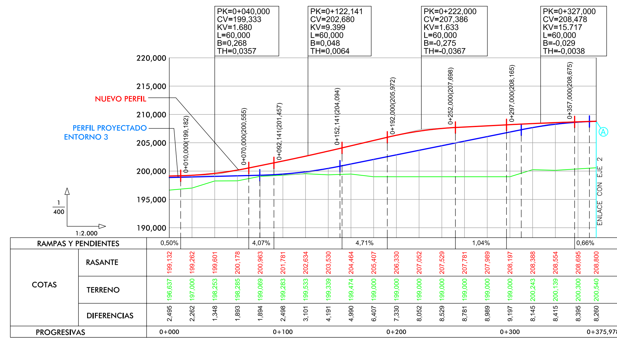
PERFIL LONGITUDINAL EJE 4a
